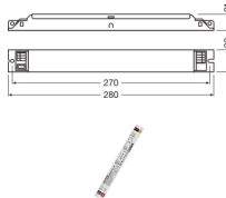
Technische Daten Osram LED driver Optotronica Fit 35 / 220-240V / 700 / CS
